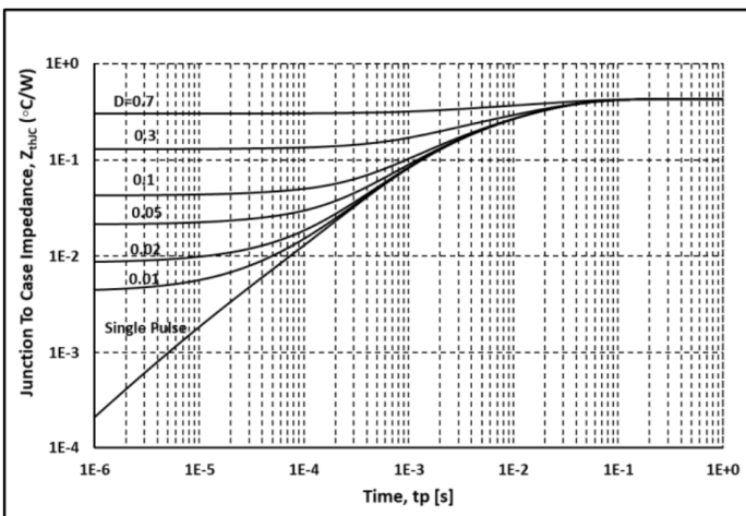
Fig. 23 Thermal Impedance
